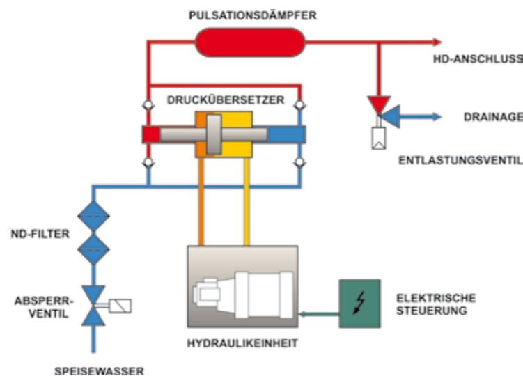
Systemschaubild der Hochdruckpumpe HYTRON®
