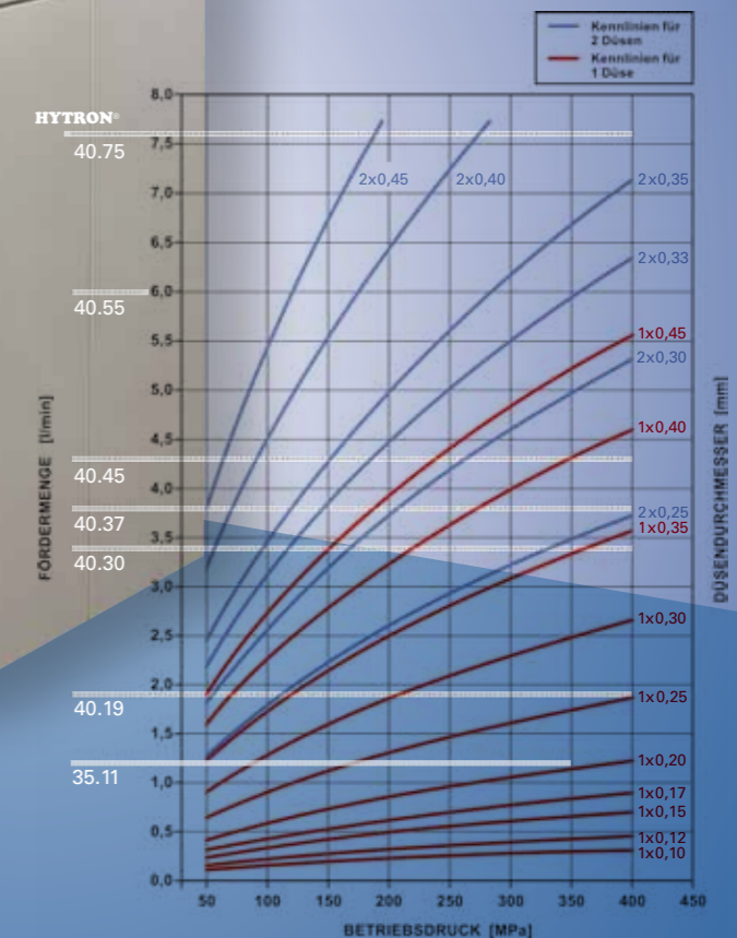
Zusammenhang zwischen Betriebsdruck, Fördermenge und Düsendurchmesser
